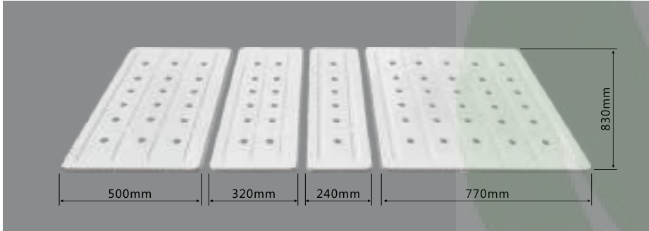
KX-505 拉伸铁床板 规格：730×315mm Size：730×315mm
